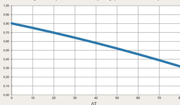
Wykres sprawności cieplnej ( G^* = 800 \text{ W/m}^2 )
