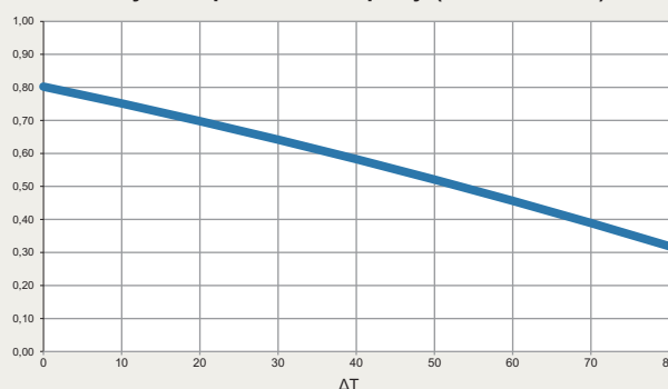
Wykres sprawności cieplnej (G* = 800 W/m 2 )
