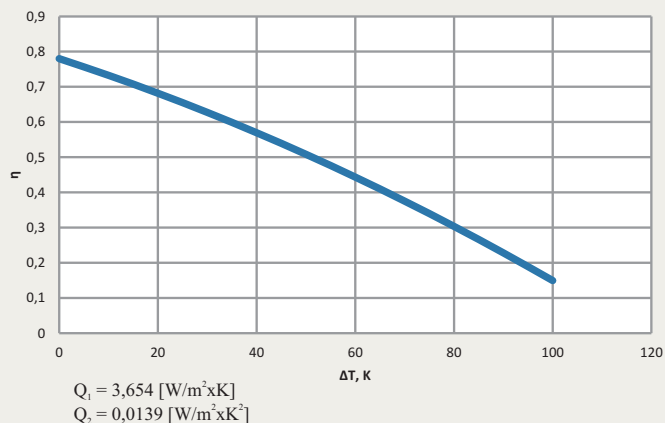
Wykres sprawności cieplnej (G* = 800 W/m2)
