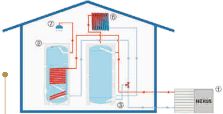
Schemat 3 Podgrzew centralnego ogrzewania i ciepłej wody użytkowej poprzez zasobnik c.w.u. i bufor c.o.
